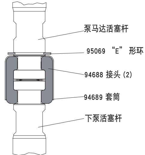
泵连接详图
